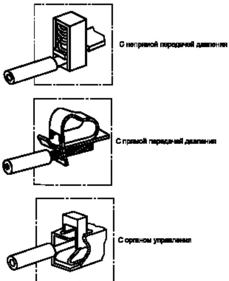
Рисунок D.7 — Безрезьбовые выводы
