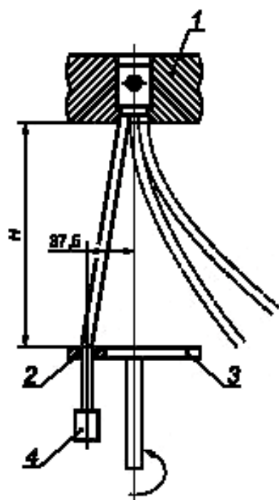
1 — узел фиксации; 2 — гильза; 3 — диск; 4 — груз
