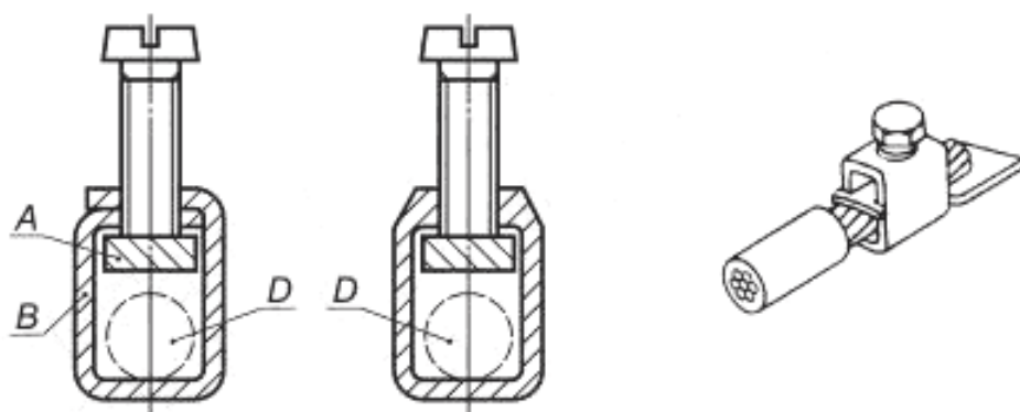
Выходы с непрямой передачей давления
