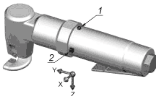
Рисунок 8 — Точки и направления измерений для ножевых ножниц для фигурной резки
