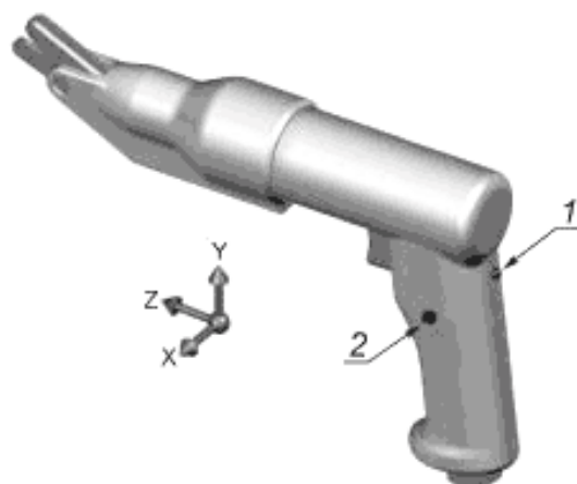
Рисунок 7 — Точки и направления измерений для ножевых ножниц с прямой рукояткой пистолетного типа
