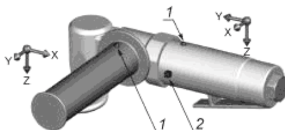
1 — предпочтительная точка измерений; 2 — дополнительная точка измерений
