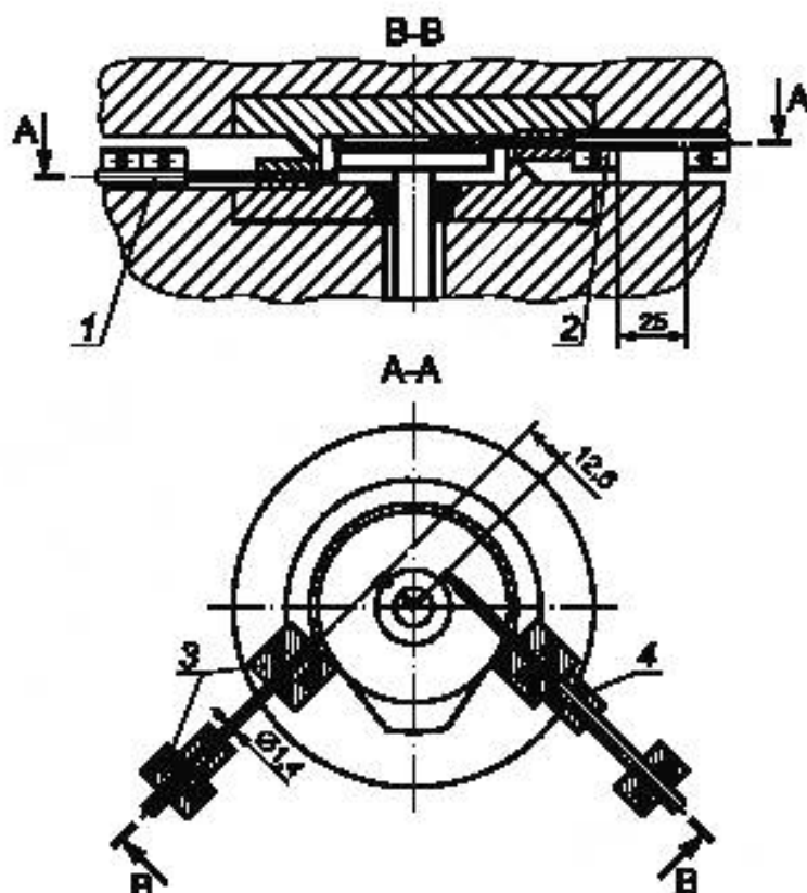
1 — удаленный измерительный зонд; 2 — вставляемый измерительный зонд; 3 — столоры, присоединенные к аппарату; 4 — столор, присоединенный к измерительному зонду
