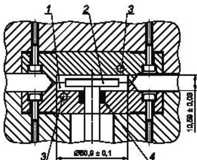
1 — камера, образуемая полуформами; 2 — ротор; 3 — датчик температуры; 4 — уплотнение
