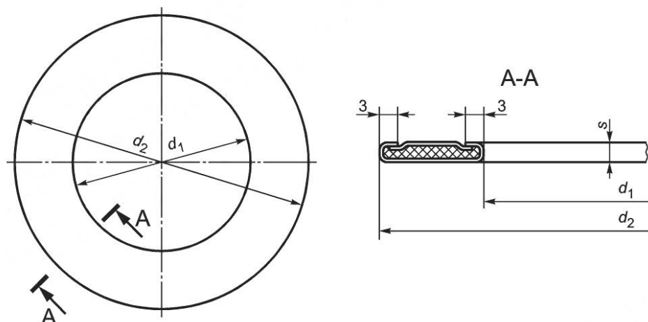
Рисунок 1 — Прокладка в металлической оболочке
