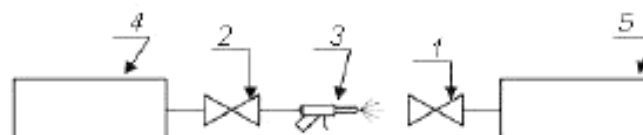
1 – испытываемый клапан, 2 – клапан, 3 – обдуватель, 4 – резервуар с пробным газом, 5 – система течеискателя
