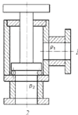
Рисунок 1 – Угловой клапан
