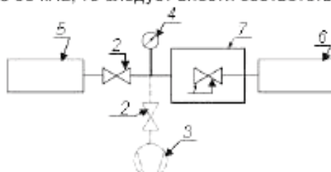
1 – испытываемый клапан, 2 – клапан, 3 – дополнительный вакуумный насос, 4 – вакуумметр, 5 – резервуар с пробным газом, 6 – система течеискателя, 7 – испытательная камера
