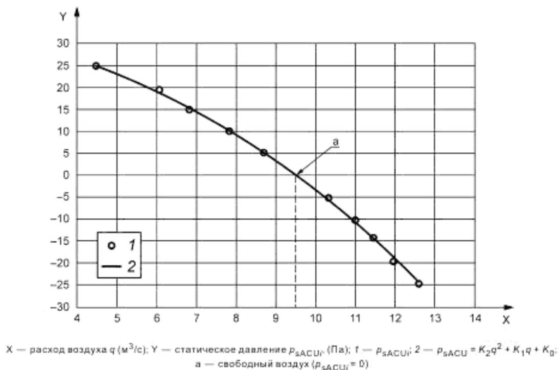
Рисунок 2 — Расход воздуха в зависимости от статического давления
