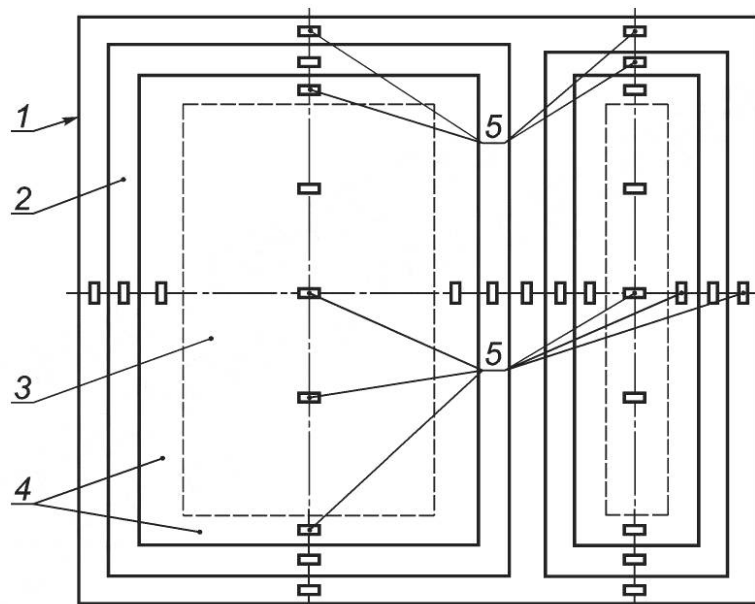
Рисунок 2 — Рекомендуемое расположение датчиков при испытании оконного блока
