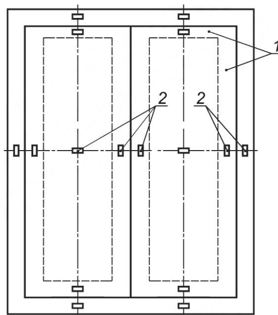
Рисунок 2 — Рекомендуемое расположение датчиков при испытании оконного блока
