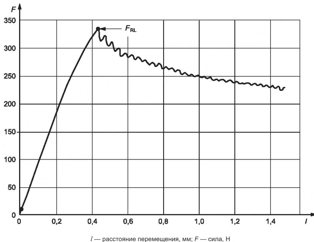
Рисунок 3 — Определение величины продольного трения F_{RL} при испытании на растяжение
