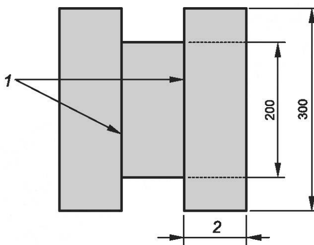
Рисунок 2 — Нарезка образцов
