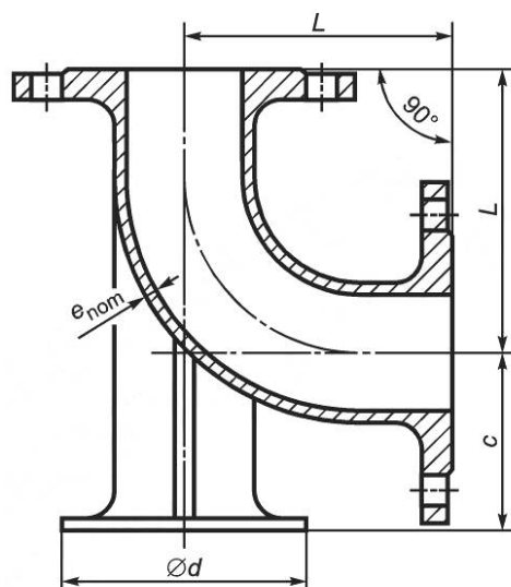
Рисунок 16 — Колено прямое лапчатое с двойным фланцем 90°
