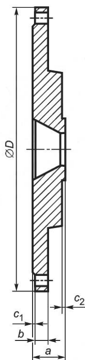
Рисунок 26 — Переходной фланец PN 25
