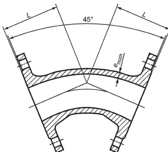
Рисунок 17 — Колено с двойным фланцем 45°
