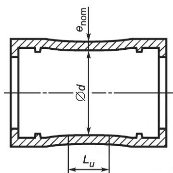
Рисунок 7 — Узкая втулка
