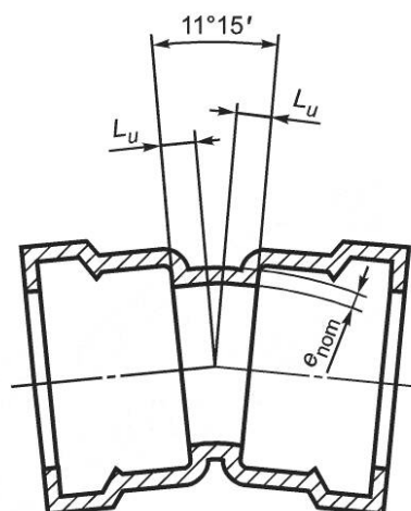
Рисунок 11 — Колено с двойным раструбом 11°15'
