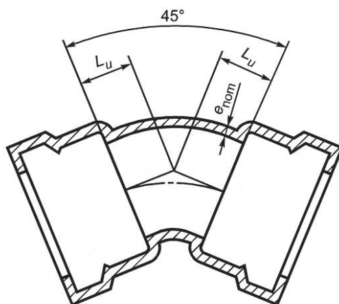
Рисунок 9 — Колено с двойным раструбом 45°
