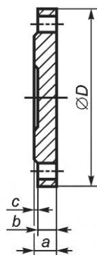
Рисунок 22 — Глухой фланец PN 25
