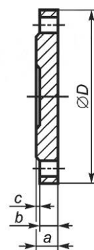
Рисунок 21 — Глухой фланец PN 16
