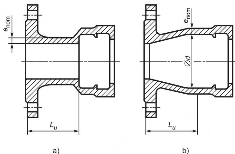
Рисунок 5 — Фланцевый растроб
