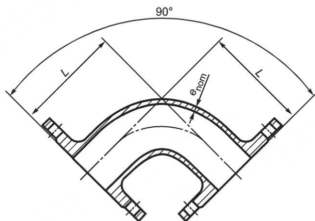
Рисунок 15 — Колено прямое с двойным фланцем 90°
