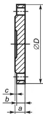
Рисунок 20 — Глухой фланец PN 10
