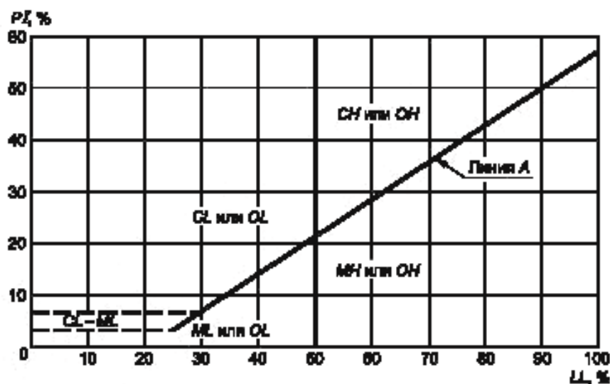
Рисунок Е.3 — График пластичности грунтов (plasticity chart)
