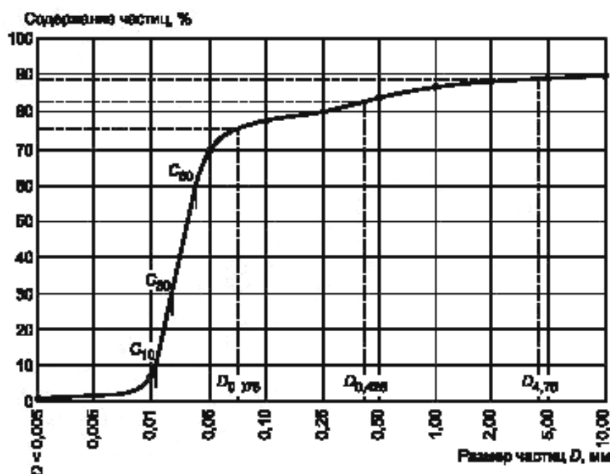
Рисунок Е.2 — Кумулятивная кривая гранулометрического состава
