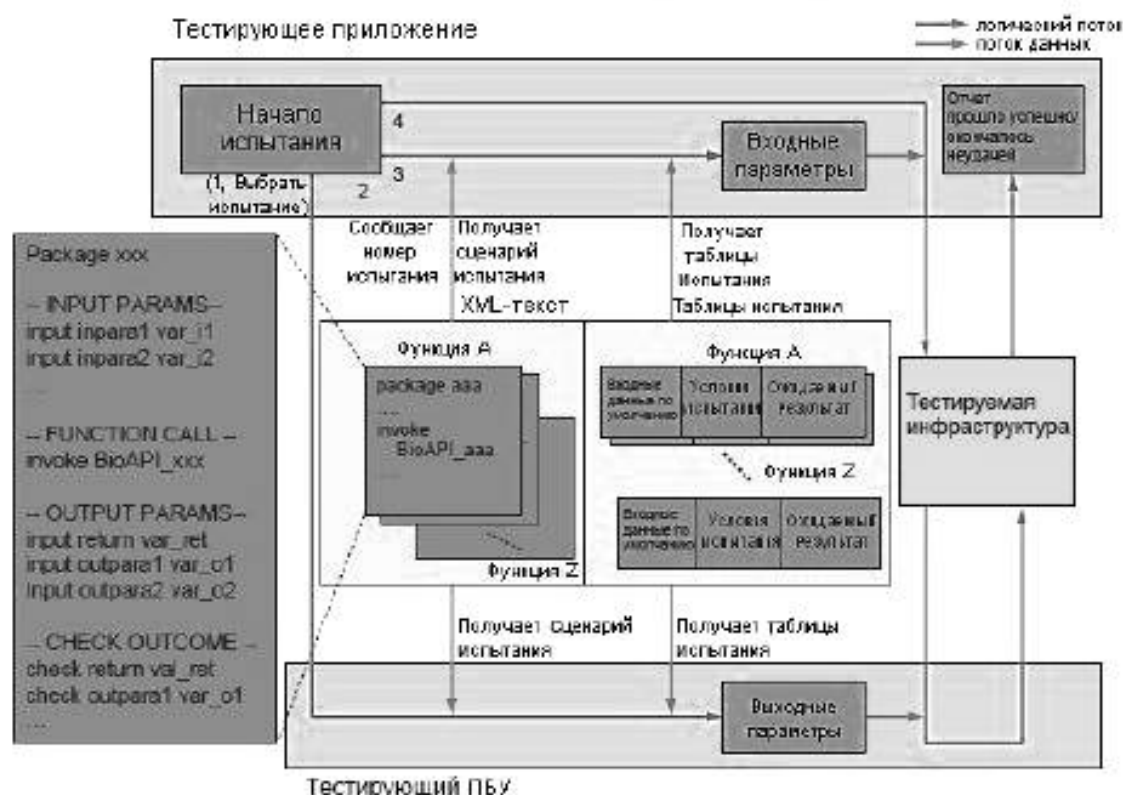
Рисунок 1 – Структура КТС для инфраструктуры БиоАПИ
