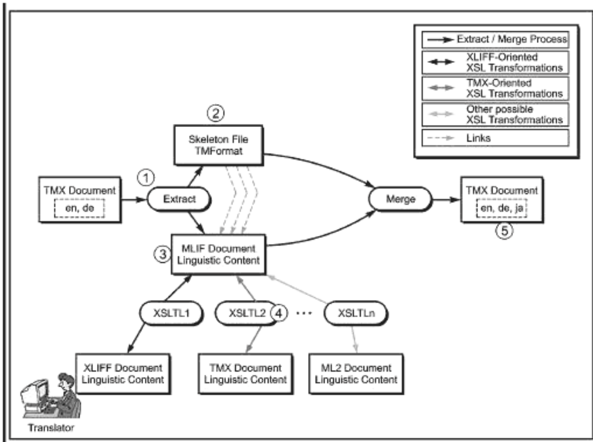
Рисунок Б.1 — Схема взаимодействия TMX и MLIF
