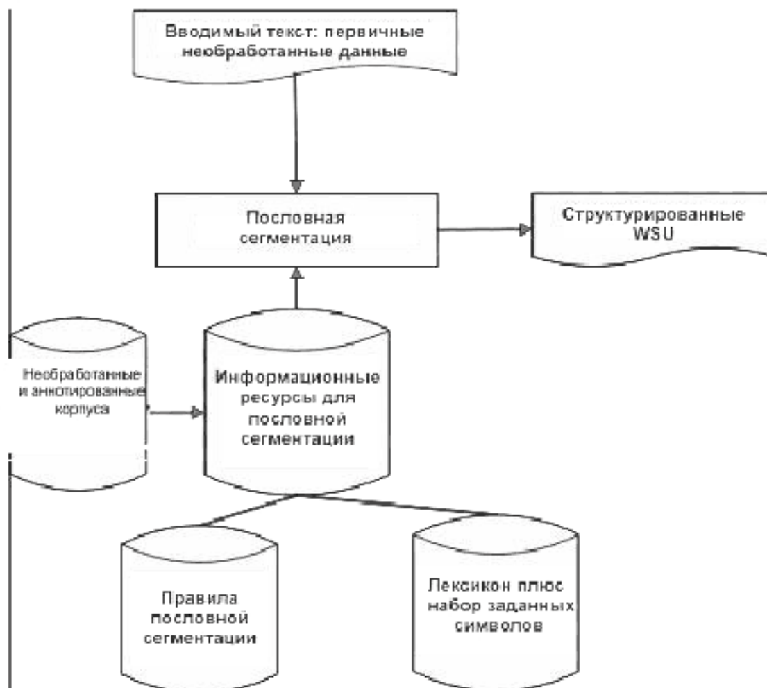
Рисунок 5. Процесс пословной сегментации
