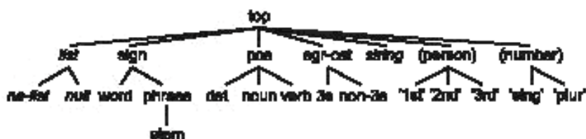
Рисунок 9 — Простая иерархия типов для английского языка
