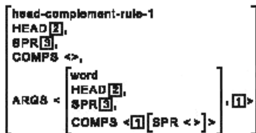
Рисунок 8 — Правило 1 для составления заголовка
