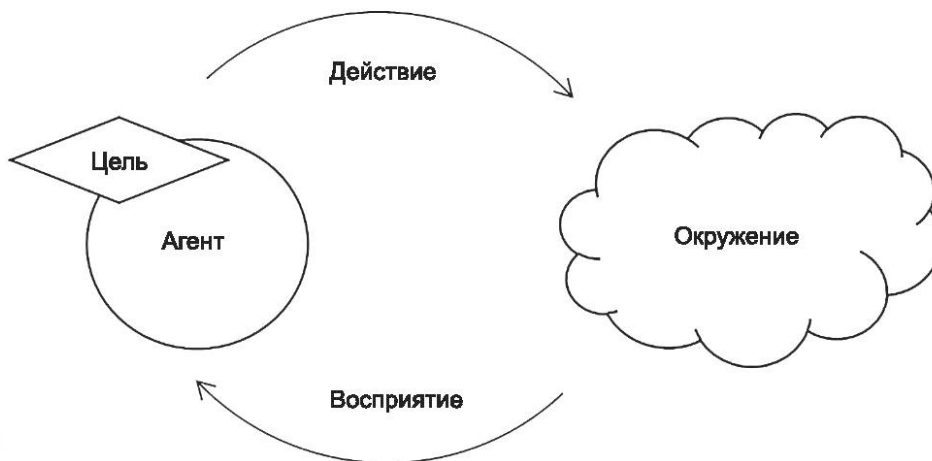
Рисунок 1 — Парадигма агента
