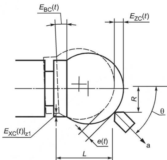
Рисунок A.5 — Общий случай погрешности перемещения
