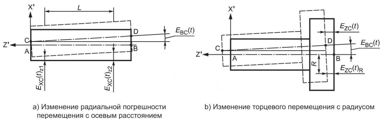
Рисунок A.4 — Геометрия радиальной погрешности перемещения и торцевого перемещения
