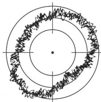
а) Общая погрешность перемещения
