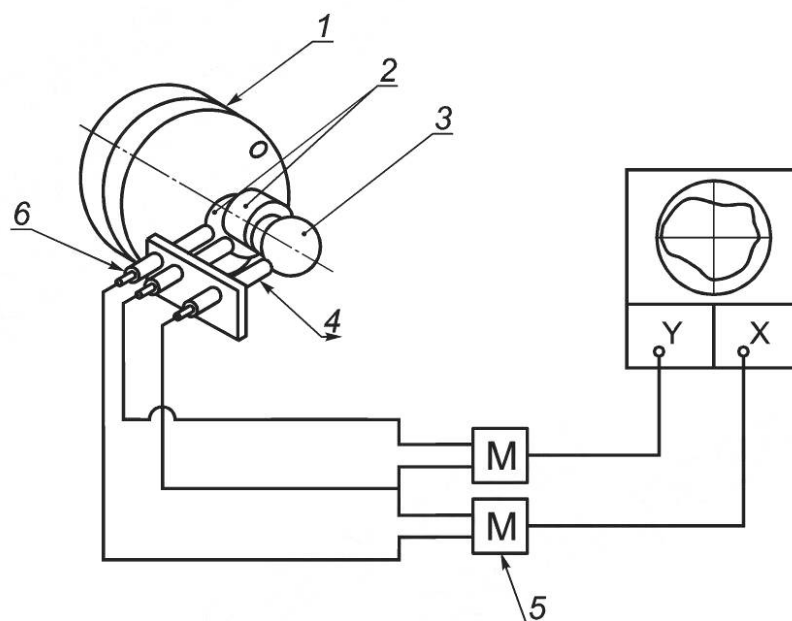
1 — колебательная плита; 2 — эксцентрированные кулачки; 3 — контрольная сфера; 4 — измерительный преобразователь перемещения; 5 — усилитель; 6 — измерительный преобразователь малого увеличения
