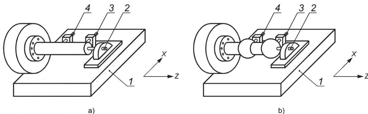
Рисунок 14 — Испытательные установки, используемые для измерения погрешности перемещения шпинделя при фиксированном чувствительном направлении
