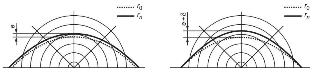
Рисунок A.14 — Влияние фундаментальной погрешности перемещения из-за структурной симметрии и асимметрии в изменяющемся чувствительном направлении
