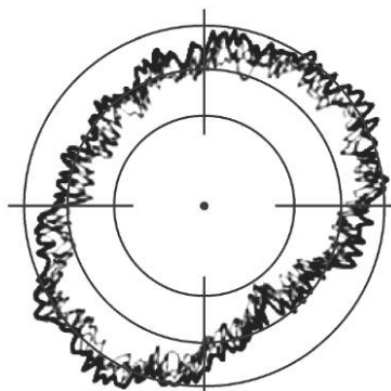
e) Внешняя погрешность перемещения
