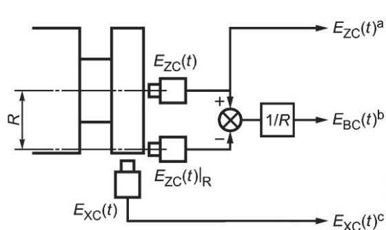
а) Испытательное устройство с использованием измерения радиальной, торцевой и осевой погрешности перемещения
