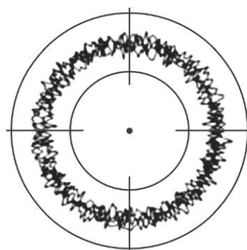
c) Асинхронная погрешность перемещения
