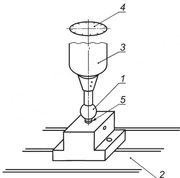
1 — контрольный объект (испытуемая сфера); 2 — стол; 3 — шпиндель; 4 — угловое измерительное устройство; 5 — измерительный преобразователь перемещения
