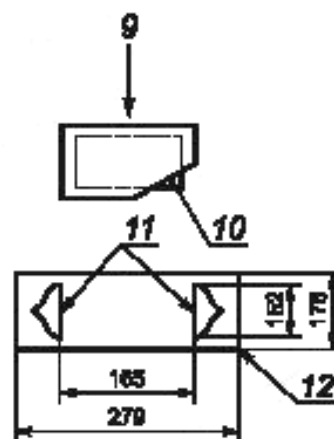
б) Схема держателя образцов для испытаний
