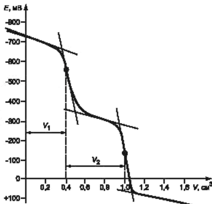
Рисунок 3 — Кривая титрования смеси сероводорода и меркаптанов
