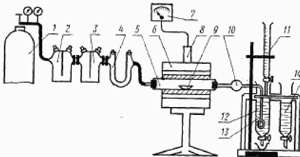
Установка для определения массовой доли серы
