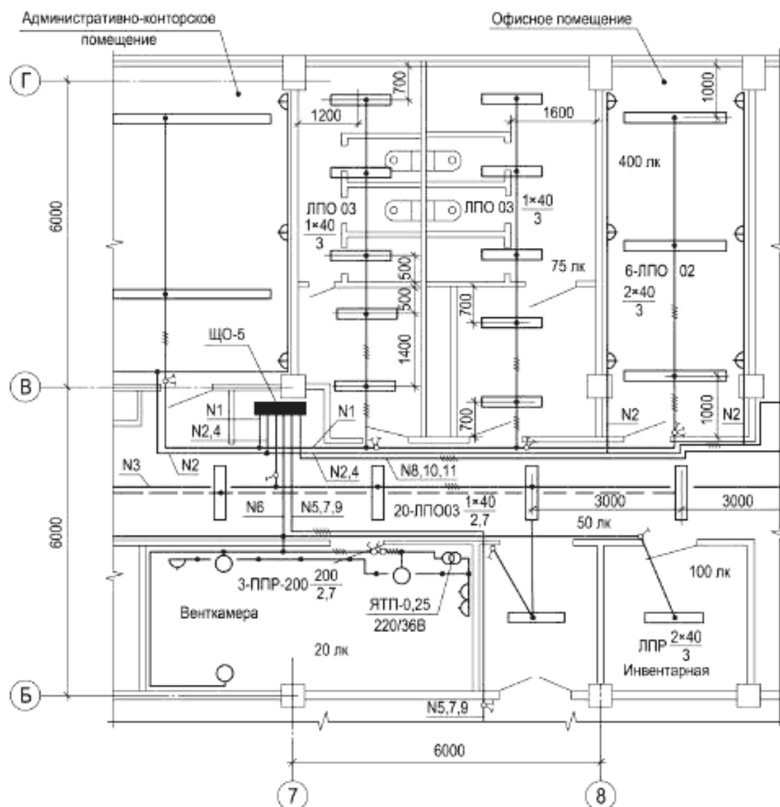
Рисунок Б.2 — Пример оформления плана расположения электрического оборудования и прокладки электрических сетей для общественного здания
