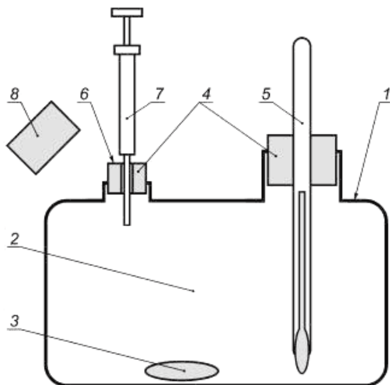
1 — стеклянная камера; 2 — насыщенные пары ртути; 3 — капля ртути; 4 — пробки из бутилкаучука; 5 — термометр; 6 — порт для отбора проб; 7 — микрошприц; 8 — крышка порта для отбора проб
