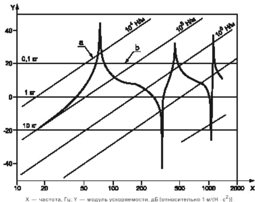
Рисунок 2 — График модуля ускорения, соответствующий графику подвижности (рисунок 1)
