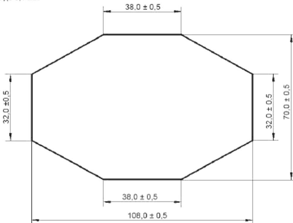
Рисунок Е.1 – Образец для определения сопротивления разрастанию трещин
