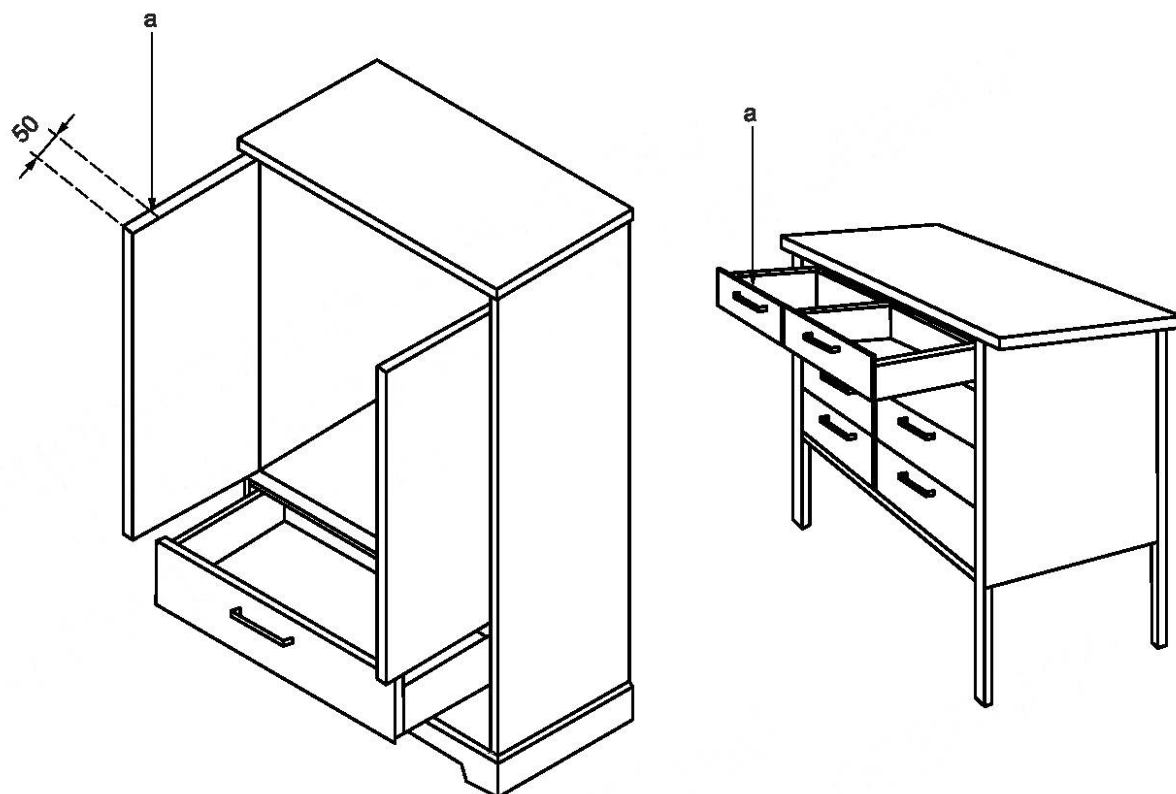
а) Вертикальная нагрузка на расстоянии 50 мм от переднего края открытой двери
