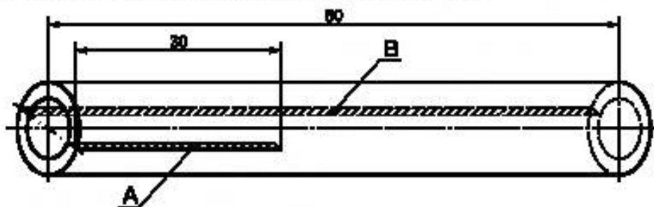
Рисунок В.1 — Размеры образца для испытаний
