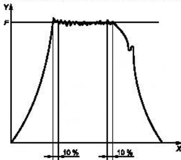
Рисунок В.3 — Типичный график определения сопротивления раздиру трубки
