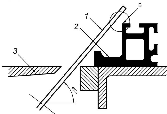
Рисунок 17 — Конструкция направляющей при установке в низкой позиции
