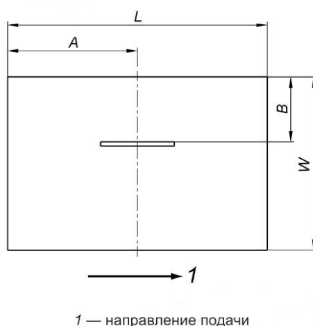
Рисунок 15 — Размеры стола станков, у которых высота пропила составляет \leq 60 мм
