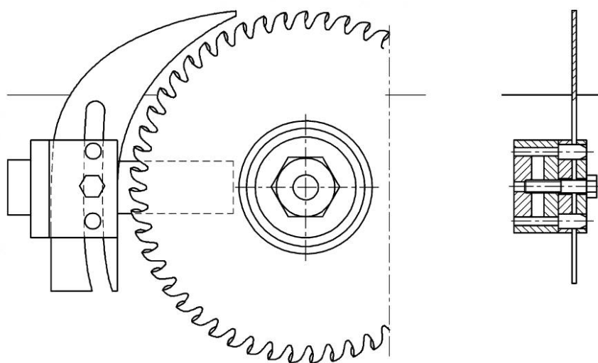
Рисунок 13 — Пример крепления расклинивающего ножа
