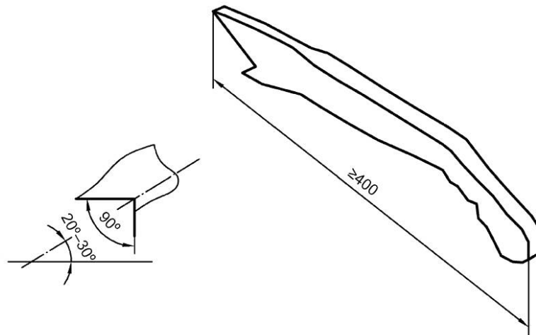
Рисунок 4 б) — Пример толкателя
