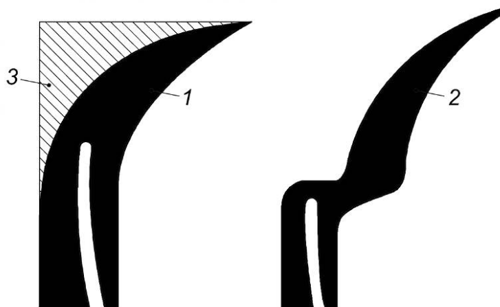
1 — пример допустимой формы расклинивающего ножа; 2 — пример недопустимой формы расклинивающего ножа; 3 — заштрихованная область показывает возможную форму расклинивающего ножа для станков с закрепленным на расклинивавшем ноже защитным ограждением
