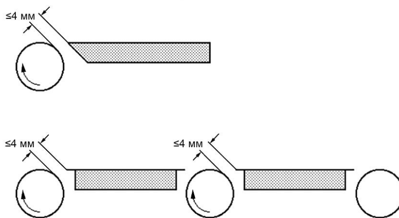
Рисунок 21 — Пример защиты стола с роликами
