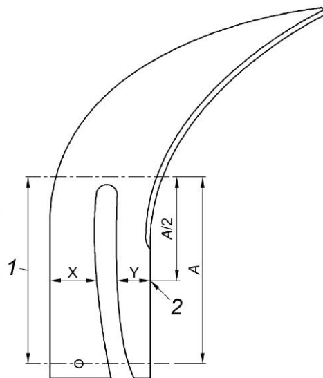
Рисунок 12 — Ширина расклинивающего ножа в области крепления
