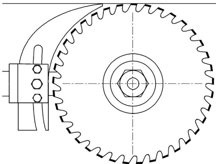
Рисунок 8 — Регулировка высоты расклинивающего ножа
