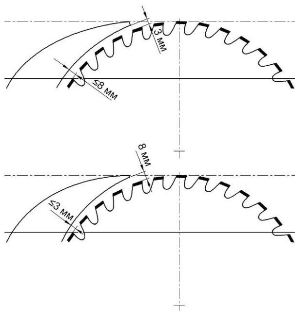
Рисунок 9 — Размеры при установке расклинивающего ножа
