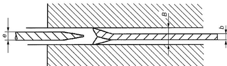
Рисунок 6 — Толщина расклинивающего ножа относительно размеров пилы
