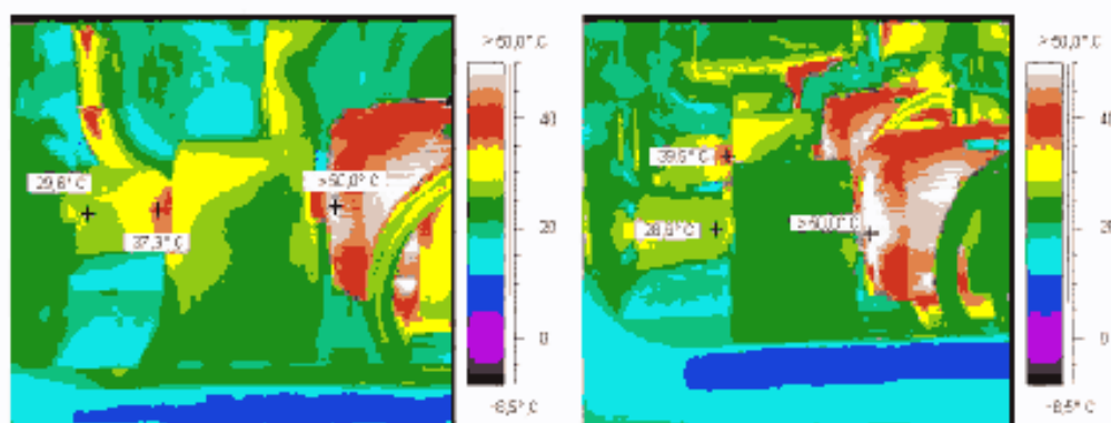
Рисунок С.9 – Термограммы насосов
