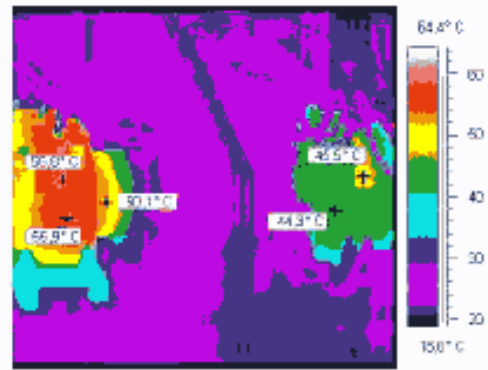
Рисунок С.7 – Корпуса подшипников шестерни привода мельницы
