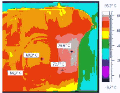
Рисунок С.5 – Редуктор со стороны двигателя
