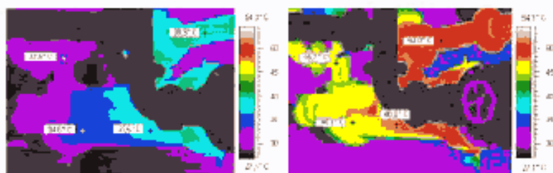
Рисунок С.10 – Термограммы двух маслоохладителей
