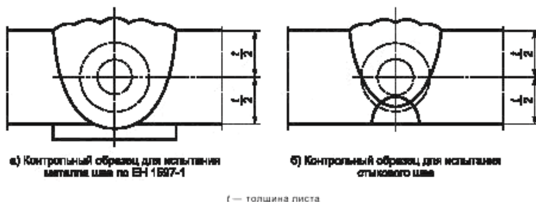
Рисунок 2 — Изготовление из контрольных образцов для испытания на растяжение металла шва
