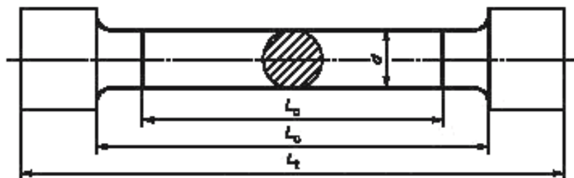
Рисунок 3 — Образец для испытания на растяжение металла шва
