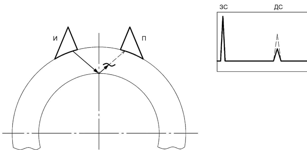
Рисунок А.6 — Зеркально-теневого метод контроля по раздельной схеме для выявления расслоений
