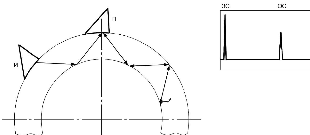
Рисунок А.4 — Эхо-импульсный метод контроля по раздельной схеме для выявления продольных дефектов
