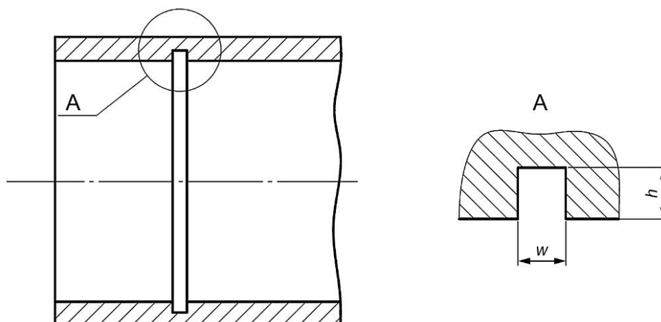
Рисунок Б.7 — Настрочный образец с кольцевым плоскодонным пазом при настройке чувствительности для выявления расслоений
