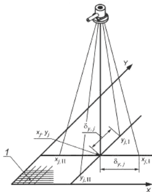
1 — пластинка с сеткой штрихов x-y
