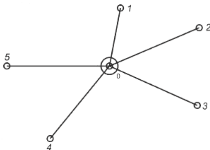
Рисунок 1 — Конфигурация для измерения горизонтальных углов
