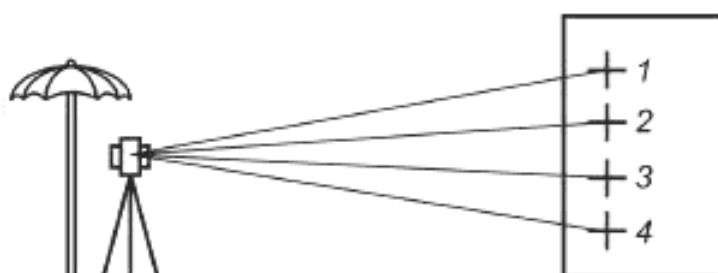
Рисунок 2 — Конфигурация для измерения вертикальных углов
