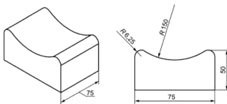
Рисунок 10 — Пример вогнутой нагрузочной подушки
