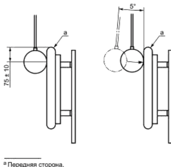
Рисунок 21 — Установка для испытания сопротивления поверхности сиденья на ударную нагрузку
