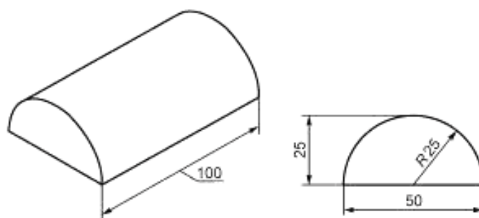
Рисунок 9 — Пример выпуклой нагрузочной подушки
