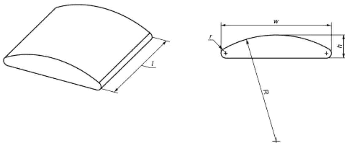
Рисунок 7 — Переменная выпуклая нагрузочная подушка
