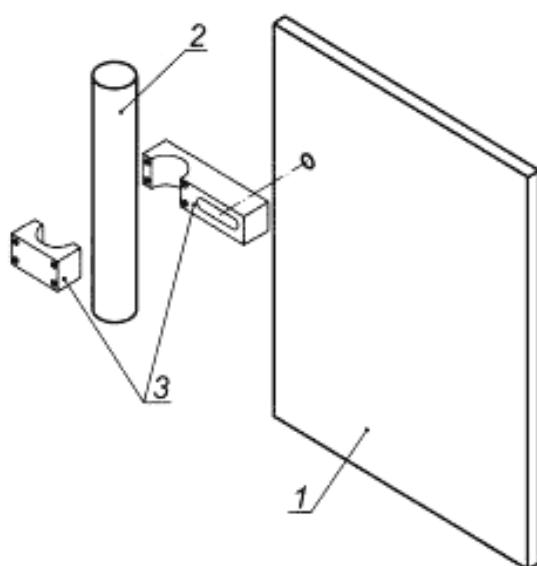
а) Установка суррогатного подсоединяемого приспособления
