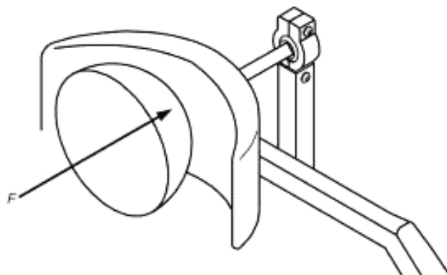
Рисунок 17 — Пример приложения задней силы к опоре головы
