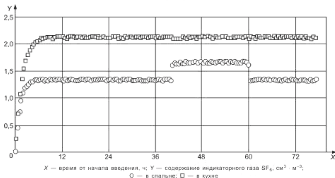
Рисунок D.5 — Результаты измерения содержания индикаторного газа с применением методики равномерного введения с активным введением и отбором проб. В период времени от 40 до 60 ч дверь в спальню была открыта (результаты моделирования)
