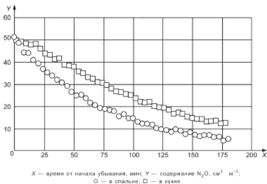
Рисунок D.1 — График зависимости содержания индикаторного газа от времени
