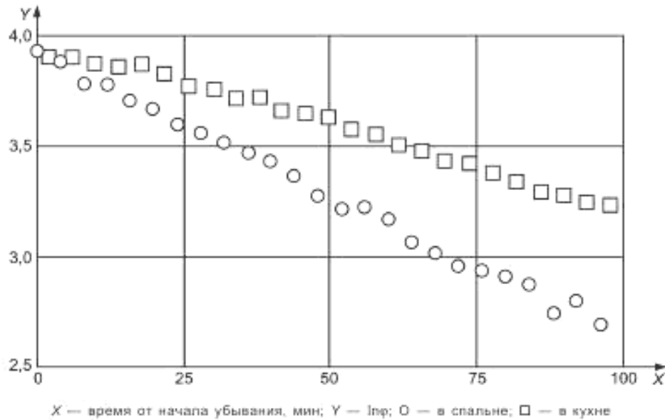
Рисунок D.2 — График зависимости логарифма содержания индикаторного газа от времени
