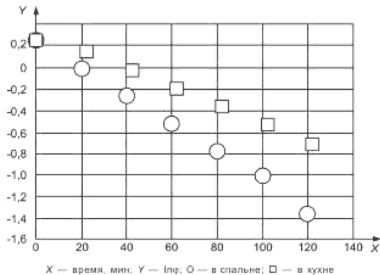
Рисунок D.3 — График зависимости логарифма содержания индикаторного газа от времени при убывании
