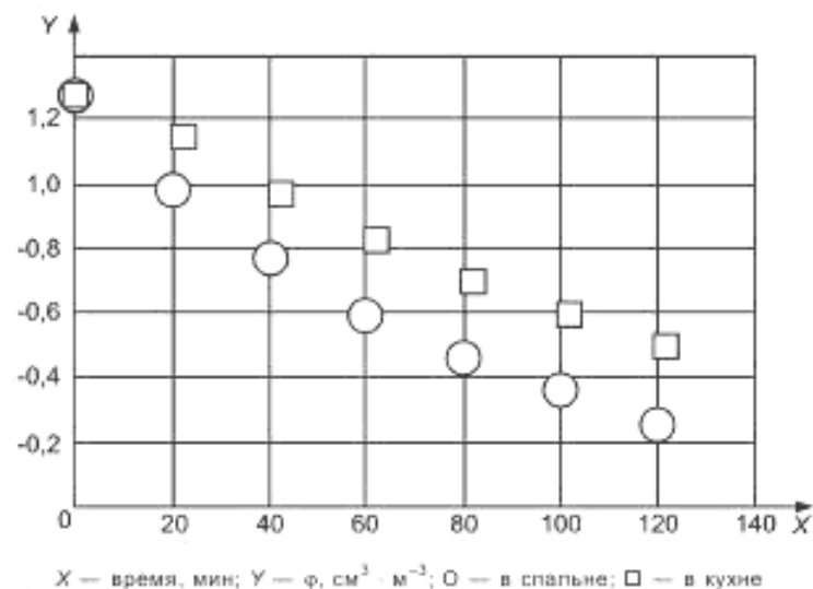
Рисунок D.4 — Линейная зависимость содержания индикаторного газа от времени при убывании
