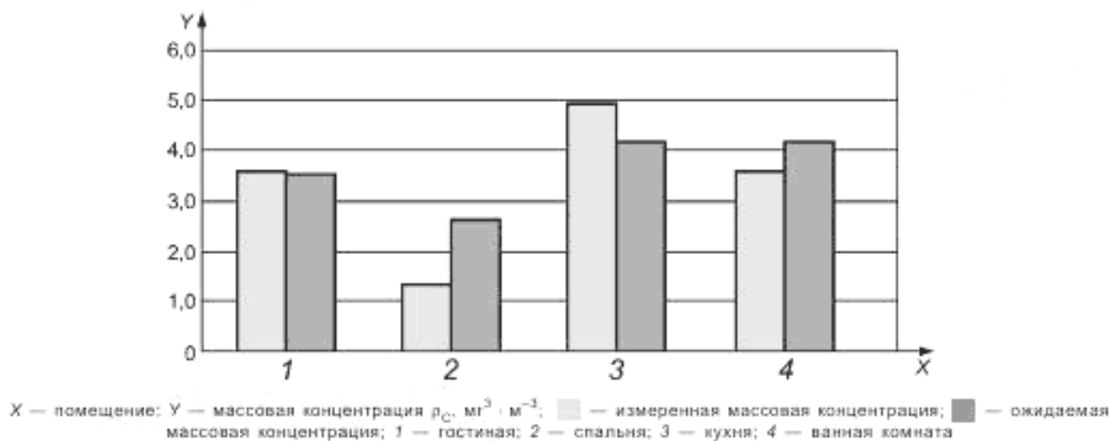
Рисунок Е.1 — Диаграмма сравнения измеренного и вычисленного ожидаемого содержания загрязняющего вещества при допущении, что при равномерном введении индикаторного газа может быть получена информация о распределении источников загрязняющего вещества
