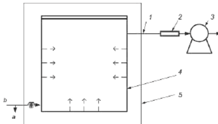
1 – передаточная линия; 2 – сорбционная трубка; 3 – побудитель расхода; 4 – микрокамера; 5 – устройство нагрева камеры; а – линия сброса избытка инертного газа; б – линия подачи инертного газа
