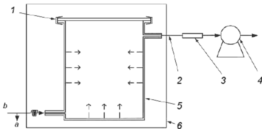
Рисунок В.2 – Схема установки для проведения испытания на выделение (первый этап испытания)
