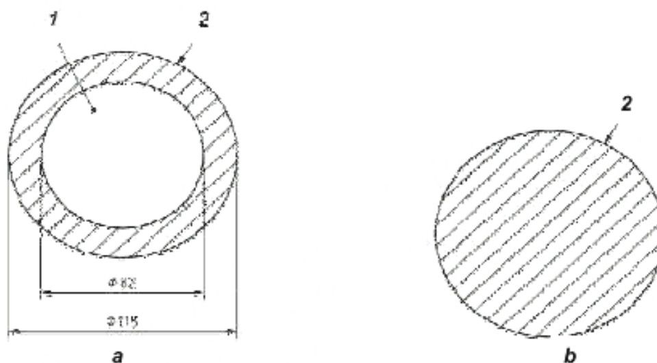
1 – исследуемая поверхность; 2 – алюминиевая фольга; а – фронтальная поверхность испытываемого образца; б – задняя поверхность испытываемого образца
