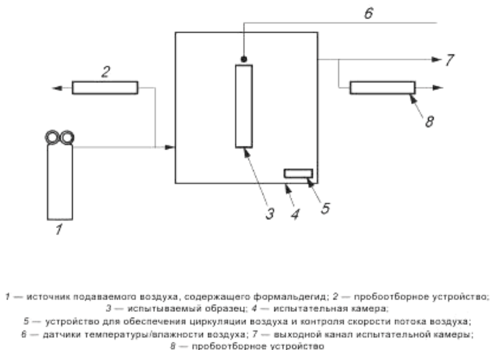
Рисунок 1 — Схема установки с испытательной камерой
