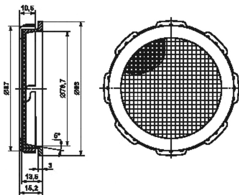
Рисунок В.2 — Одноразовый фильтродержатель
