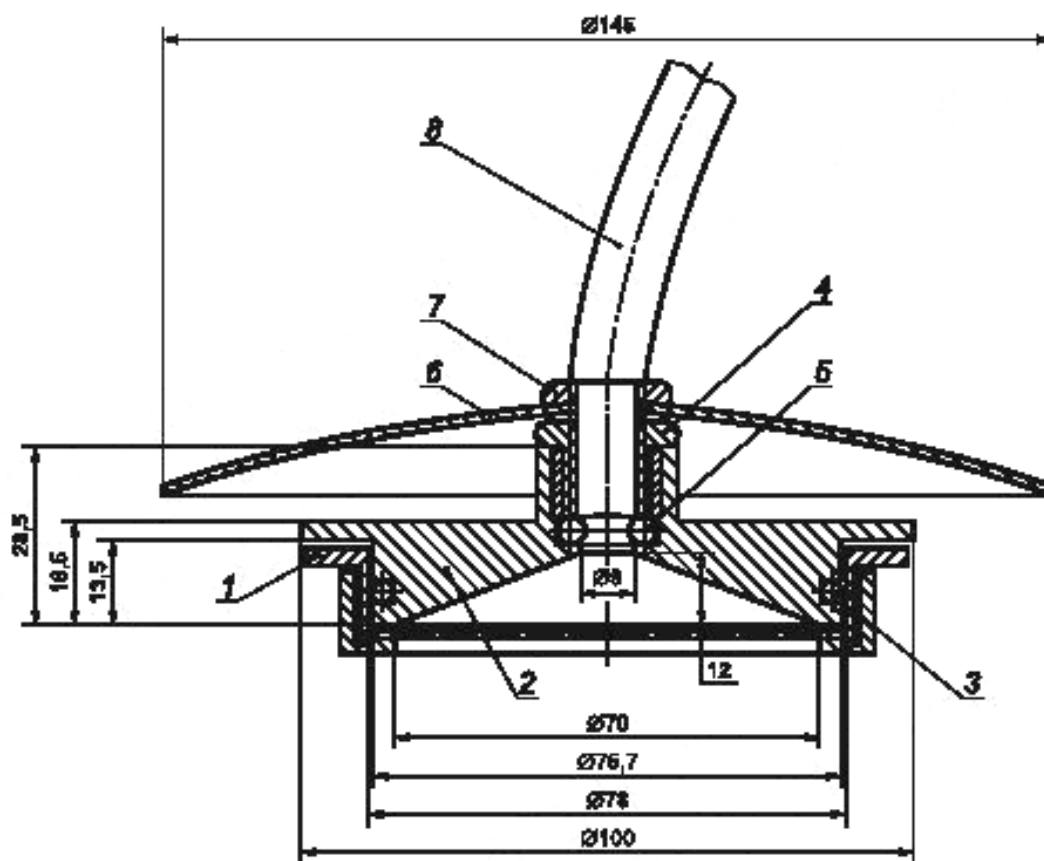
Рисунок В.1 — Пробоотборная насадка с фильтродержателем
