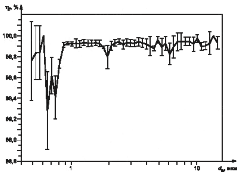
Рисунок A.2 — Характеристические кривые фильтрации для поликарбонатных фильтров (номинальной толщиной фильтрации 0,8 мкм; диаметром 80 мм) при расходе воздуха 3 м³/ч — приведенные значения получены при линейной скорости потока воздуха через фильтр v = 217 мм/с
