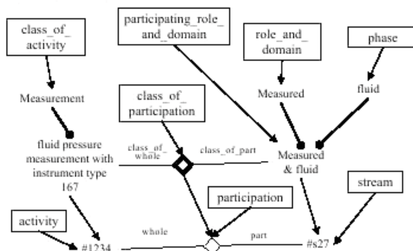
Рисунок 150 — Измерение давления флюида прибором типа 167
