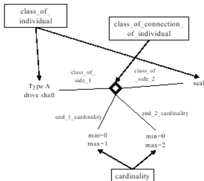
Рисунок 73 — Ограничения для классов взаимоотношения
