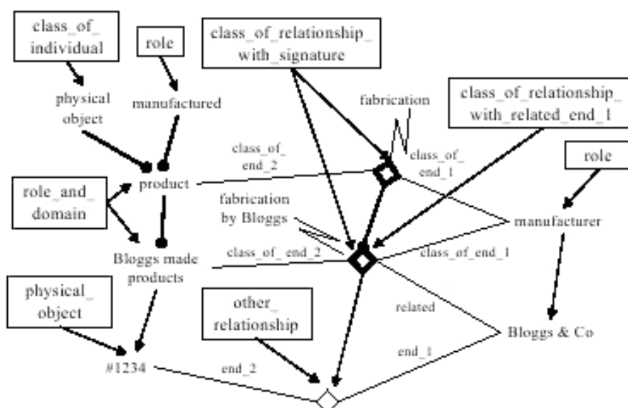
Рисунок 175 — Асимметричный класс взаимоотношения с сигнатурой
