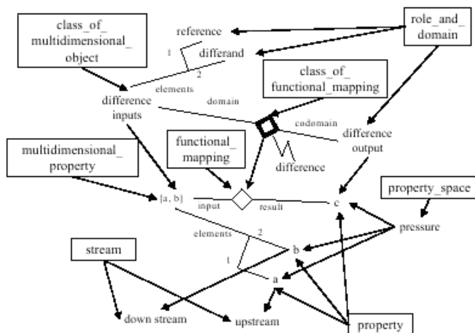
Рисунок 164 — Функциональное отображение « X^2 »
