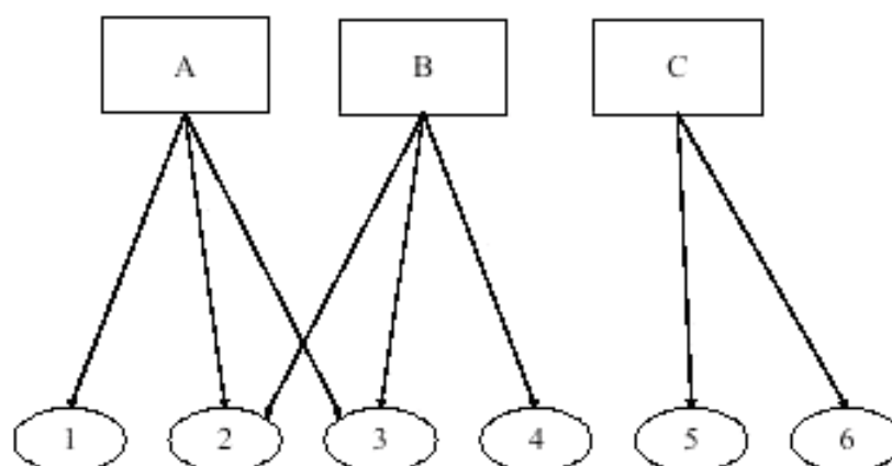
Рисунок D.1 — Одноуровневые множества
