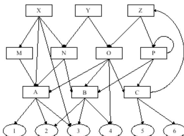
Рисунок D.4 — Пример недостаточно обоснованных множеств
