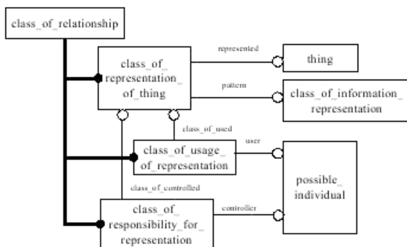
Рисунок 94 — Использование и контроль представления
