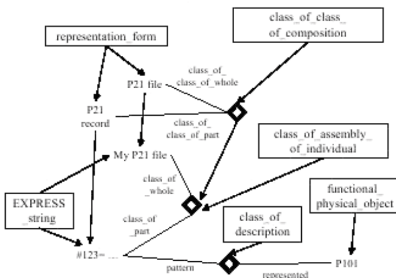
Рисунок 97 — Класс класса отображения информации
