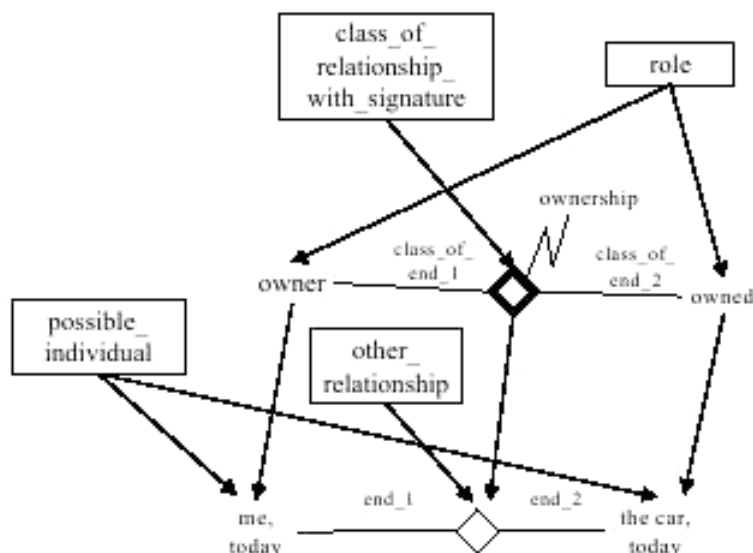
Рисунок 171 — Класс взаимоотношения с сигнатурой
