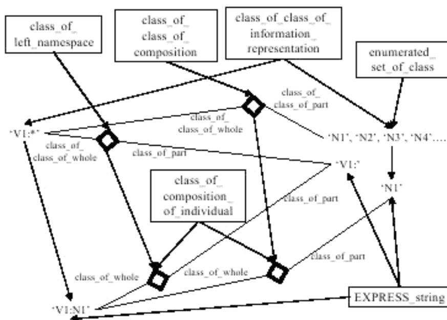
Рисунок 101 — Класс пространства имен
