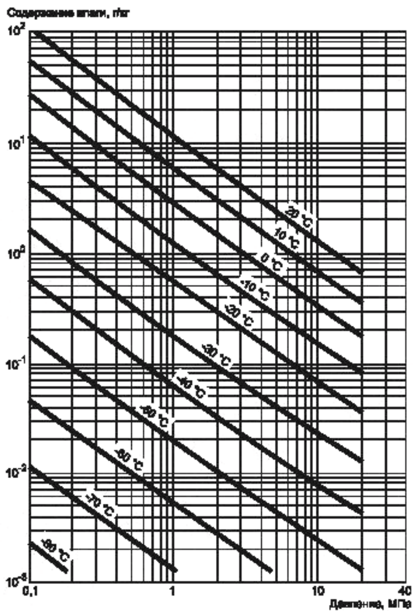
Рисунок В.2 — Диаграмма для гелия
