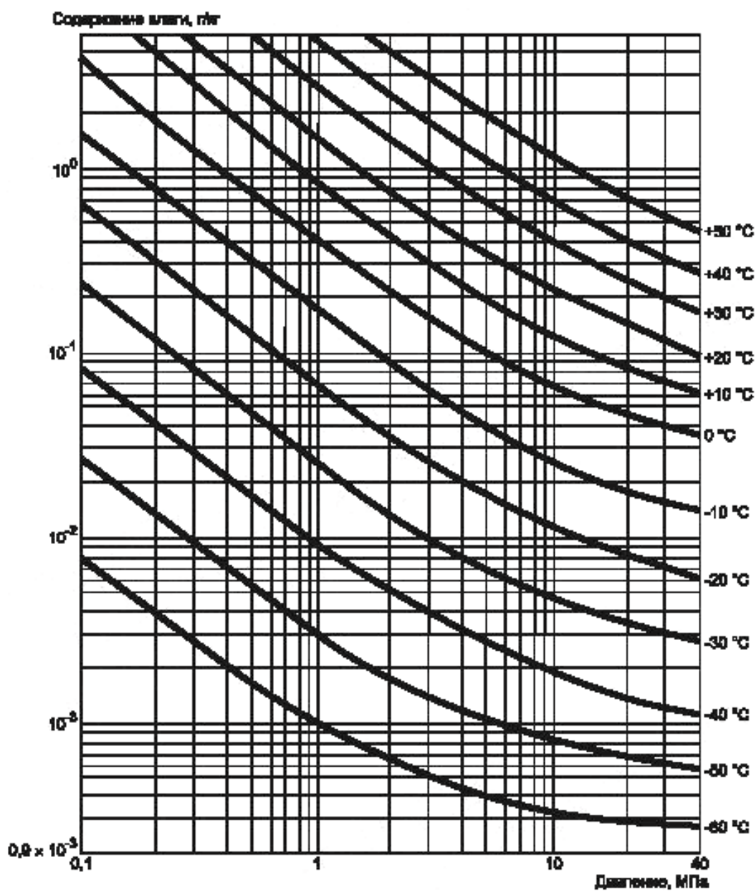
Рисунок В.1 — Диаграмма для воздуха и азота
