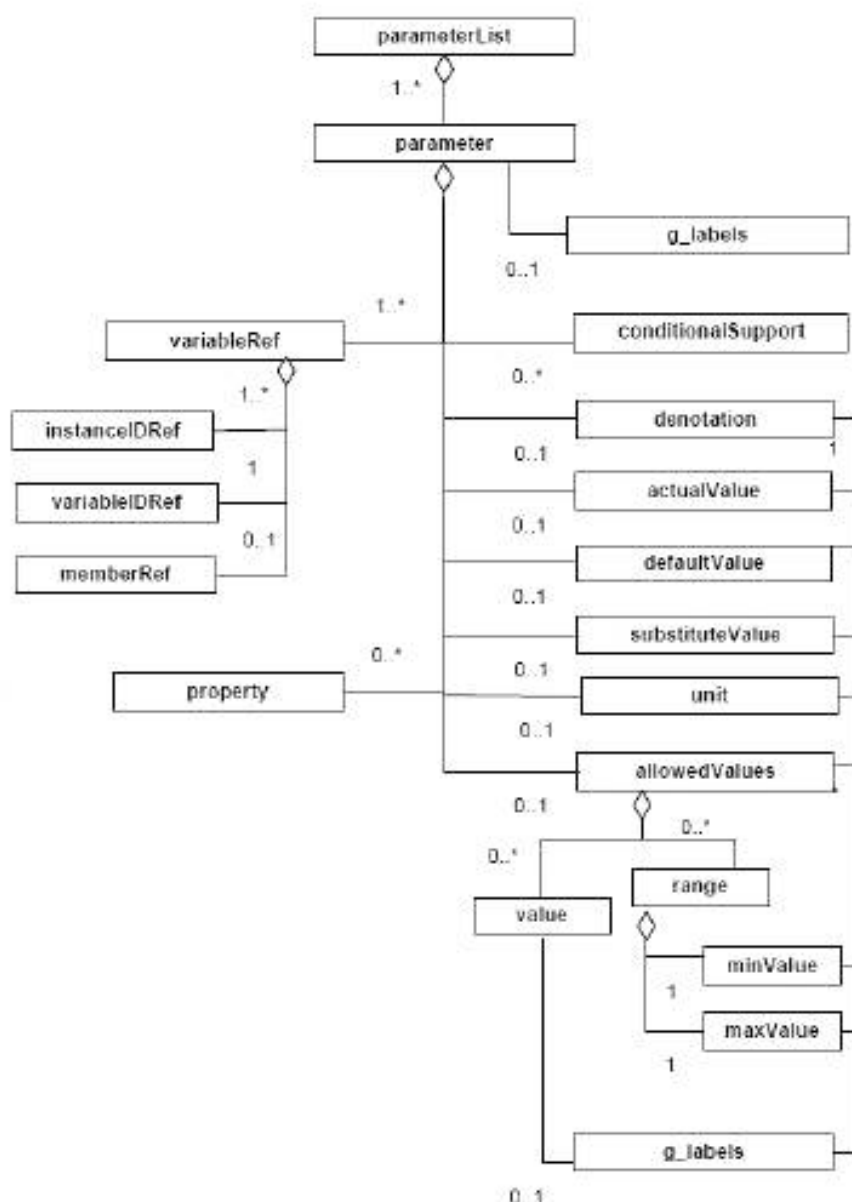
Рисунок E.7 — parameterList (список параметров)
