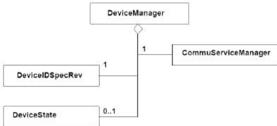
Рисунок 6 — Диаграмма класса FL-net DeviceManager
