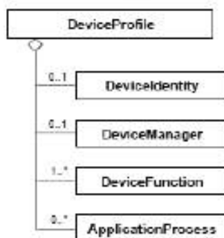
Рисунок 32 — Диаграмма класса профиля устройства ETHERNET Powerlink
