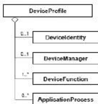
Рисунок 26 — Диаграмма класса профиля устройства EtherCAT
