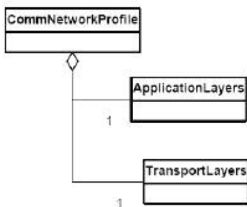
Рисунок 19 — Диаграмма класса профиля коммуникационной сети PROFINET
