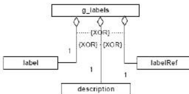
Рисунок G.2 — Группа g_labels
