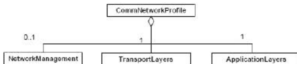
Рисунок 25 — Диаграмма класса профиля коммуникационной сети Modbus TCP
