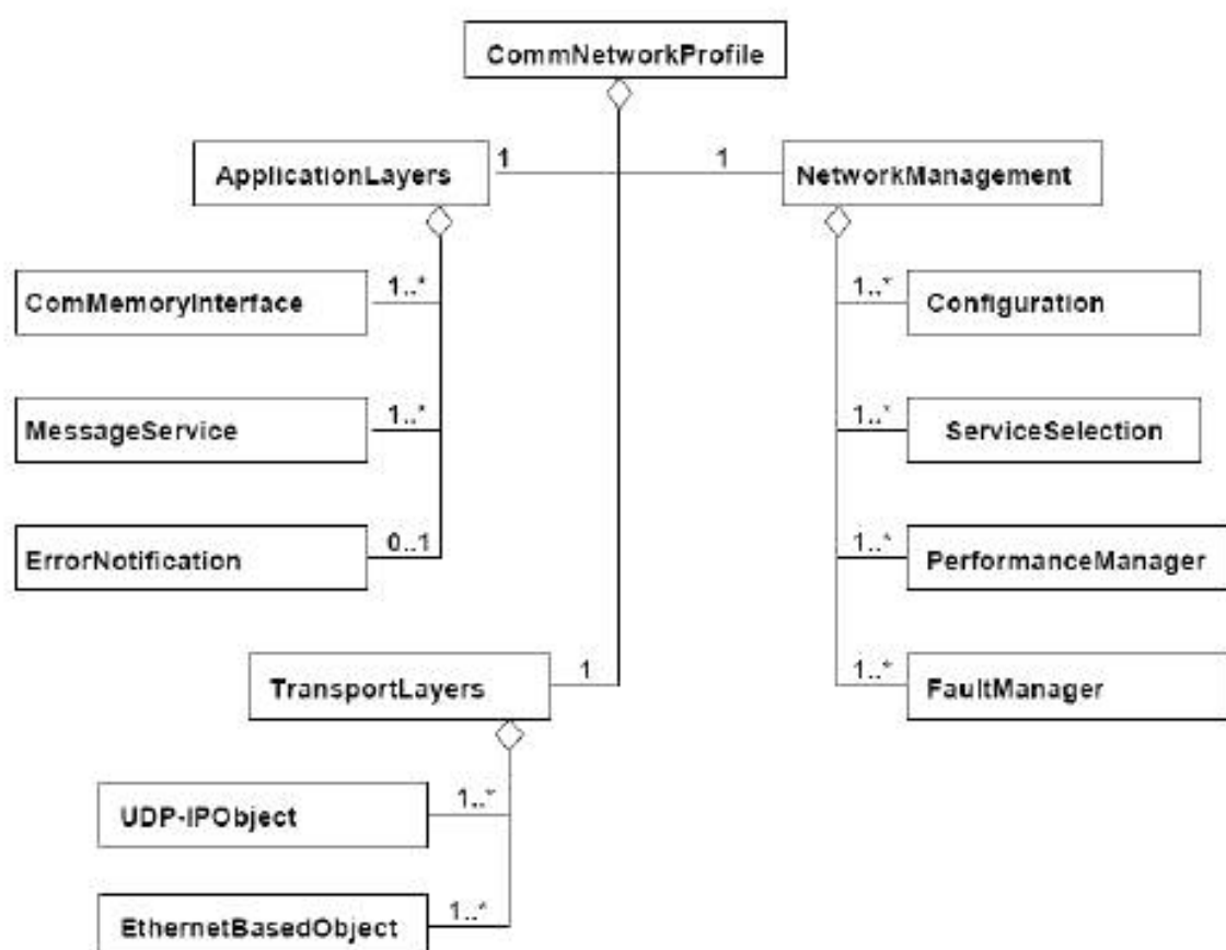
Рисунок 7 — Диаграмма класса профилей коммуникационной сети FL-net
