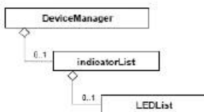
Рисунок 34 — Диаграмма класса ETHERNET Powerlink DeviceManager
