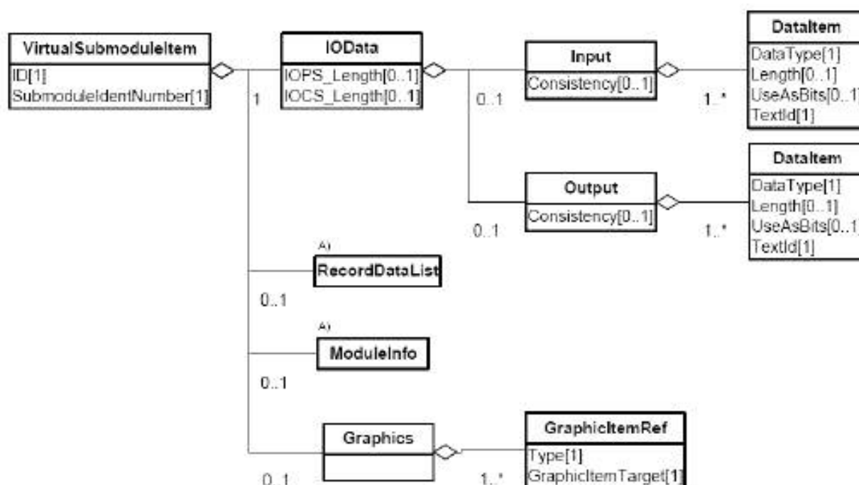
Рисунок 16 — Диаграмма класса PROFINET VirtualSubmoduleItem
