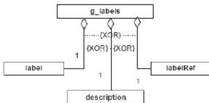
Рисунок Е.2 — Группа g_labels
