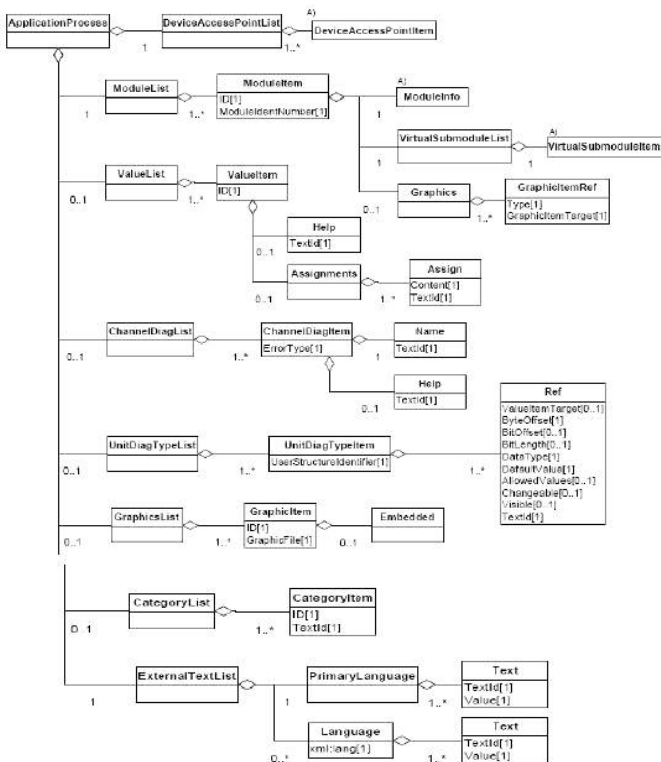
Рисунок 14 — Диаграмма класса ApplicationProcess PROFINET
