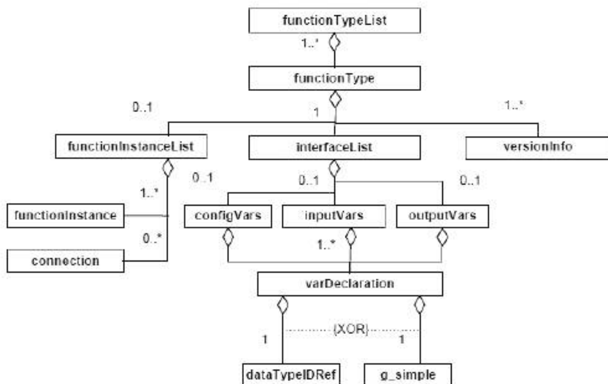
Рисунок Е.6 — functionTypeList (список типов функций)
