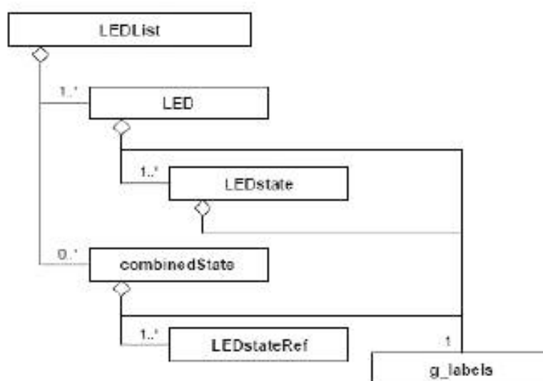
Рисунок G.4 —LEDList (LED список)
