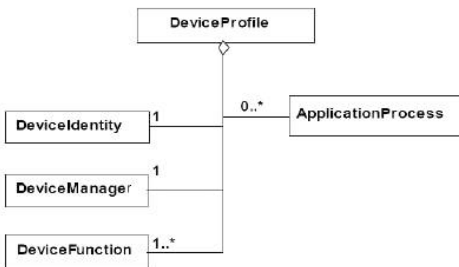
Рисунок 4 — Диаграмма класса профиля устройства FL-net
