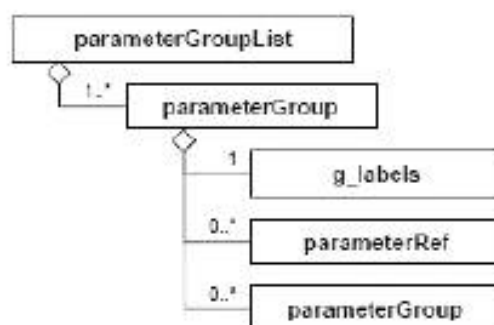
Рисунок F.8 — parameterGroupList (список группы параметров)
