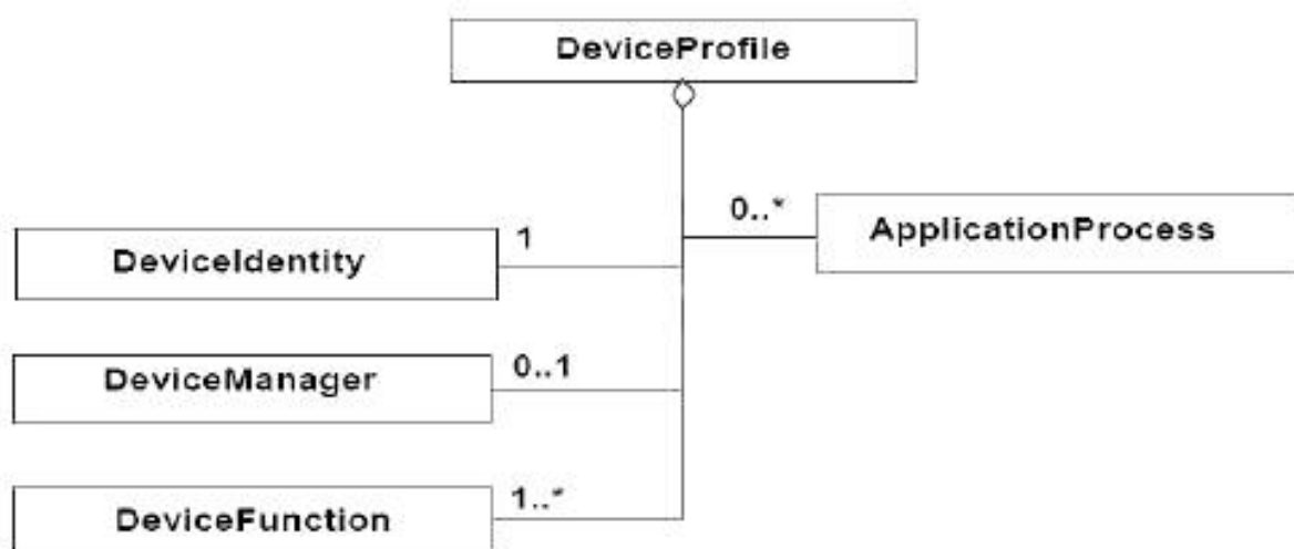
Рисунок 1 — Диаграмма класса профилей устройства ADS-net
