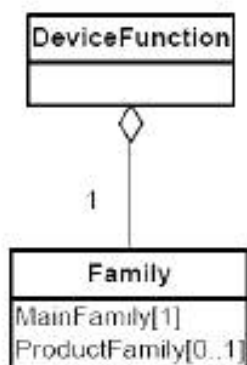
Рисунок 13 — Диаграмма класса DeviceFunction
