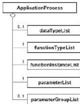
Рисунок 30 — Диаграмма класса EtherCAT Application Process
