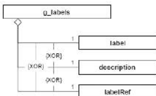
Рисунок F.2 — Группа g_labels
