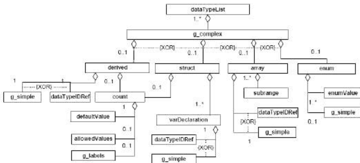
Рисунок Е.5 — dataTypeList (список типов данных)
