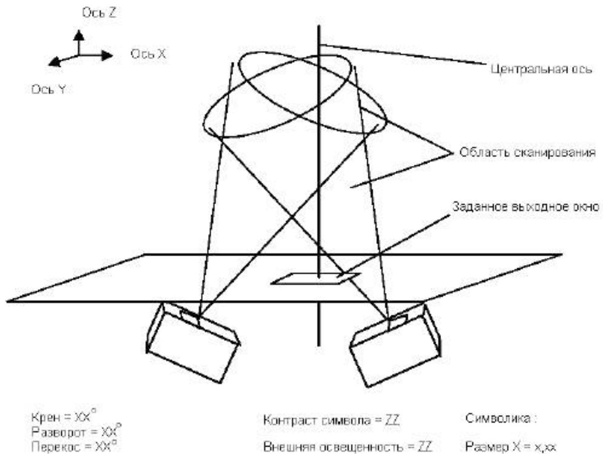
Рисунок В.5 – Диаграмма многооконного сканера
