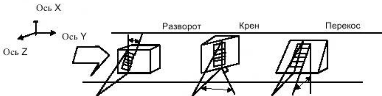
Рисунок 1 – Углы считывания
