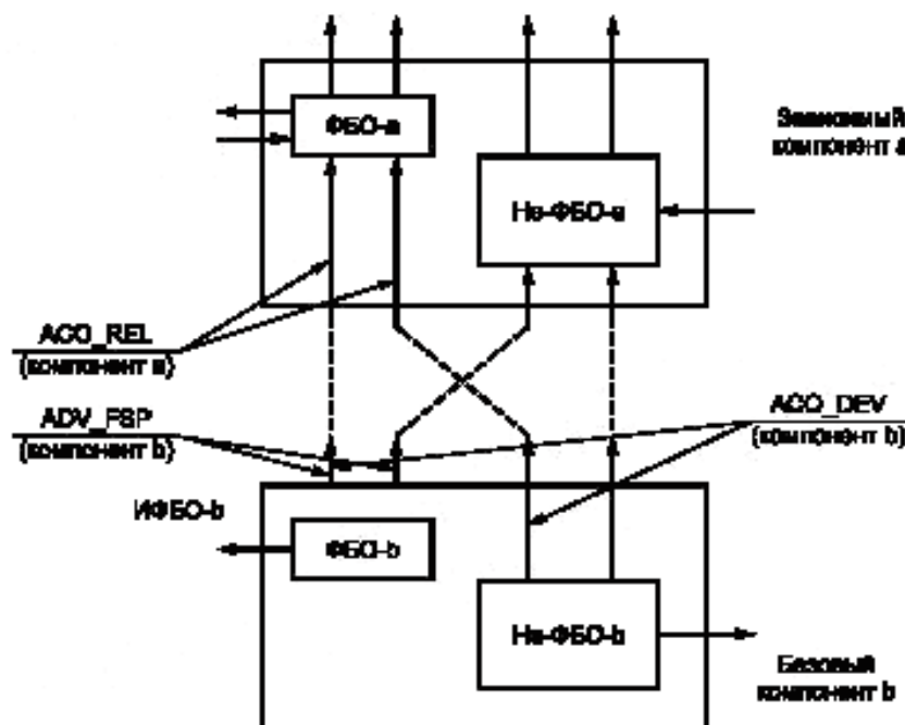
Рисунок 16 — Взаимосвязь между семействами АСО и взаимодействиями между компонентами
