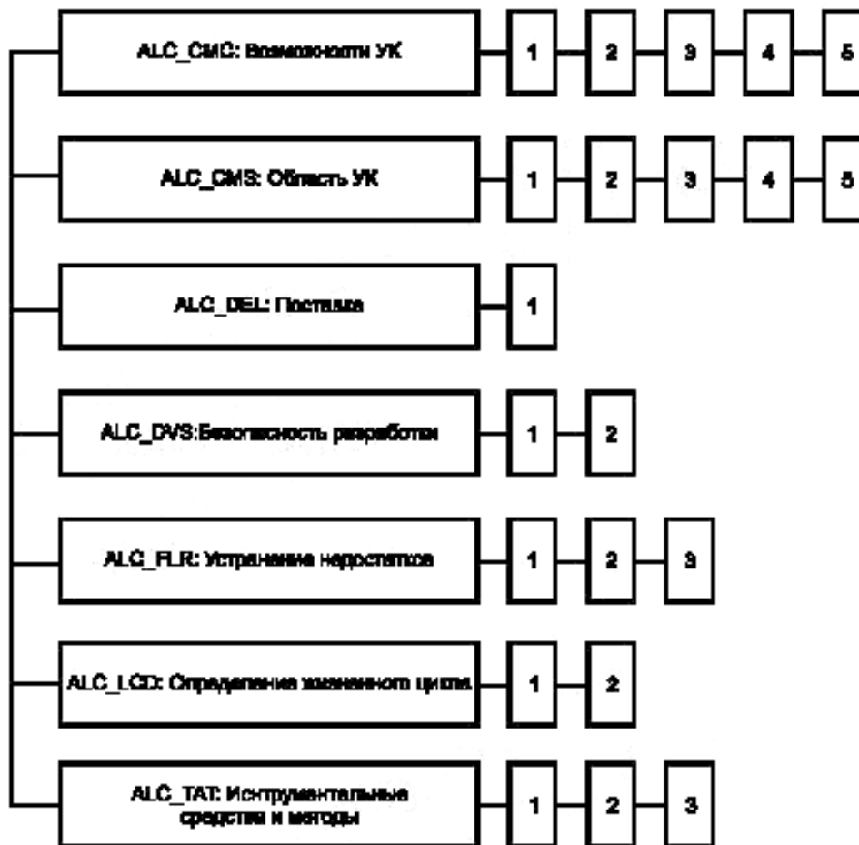
Рисунок 13 — Декомпозиция класса ALC «Поддержка жизненного цикла»
