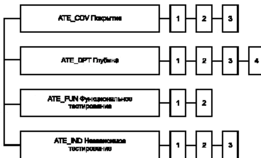
Рисунок 14 — Декомпозиция класса ATE «Тестирование»
