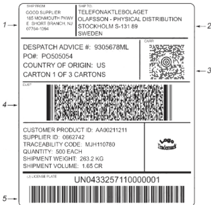
1 — отправитель; 2 — получатель; 3 — двумерный символ для сортировки/отслеживания движения и мест нахождения груза перевозчиком; 4 — двумерный символ с данными получателя или заказчика; 5 — уникальный идентификатор транспортируемой единицы в символе Code 39 с идентификатором данных J
