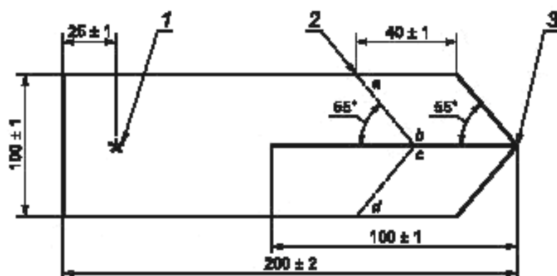
Рисунок 1 — Испытуемый образец в форме крыльев
