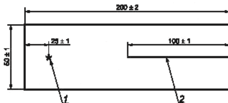
Рисунок 1 — Испытываемый образец в форме брюк
