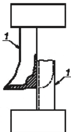
Рисунок D.2 — Зажим испытываемых образцов в зажимных устройствах
