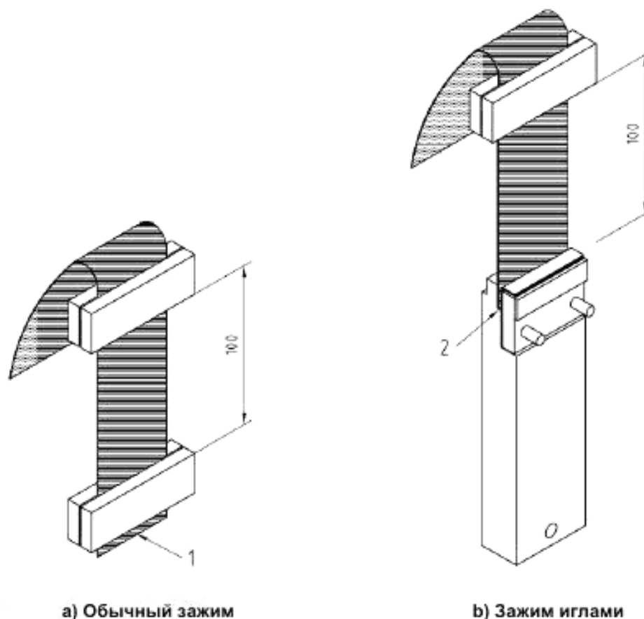
Рисунок 2 – Положение образца для испытаний
