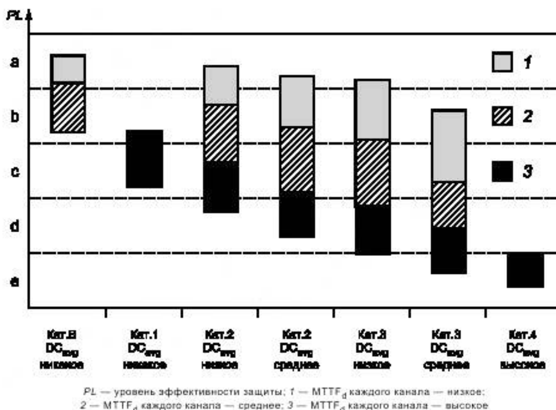
Рисунок 5 — Отношения между категориями DC_{avg} , MTTF_d каждого канала и PL
