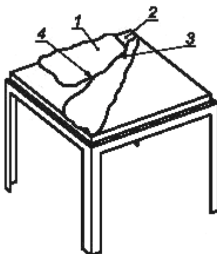
1 — подушка (размер половины масштаба); 2 — положение нижней простыни; 3 — верхнее покрывала (одеяла), отогнутые под углом примерно 30 °С; 4 — источник пламени, размещенный по центру соединения между нижней простыней и откинутыми верхними покрывалами (одеялами)
