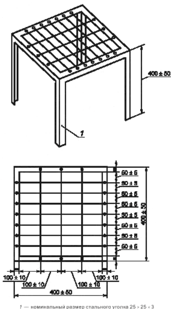
Рисунок 1 — Испытательный стенд
