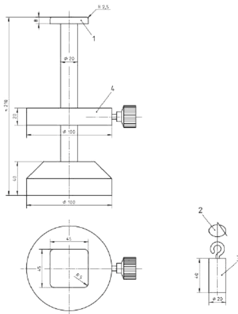
1 – монтажный столик; 2 – зажим; 3 – груз; 4 – опускающаяся консоль
