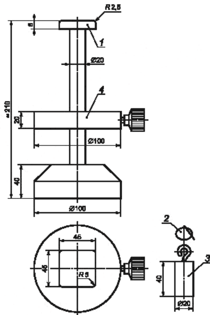
Рисунок А.1 — Монтажное приспособление для облегчения подготовки высокоэластичных полотен
